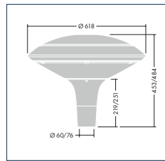
CHAPEAU DISC Ø 60 & Ø 76
