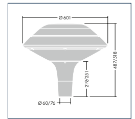
CHAPEAU FLAT Ø 60 & Ø 76
