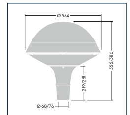
CHAPEAU ROND Ø 60 & Ø 76
